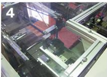
4 1時間当たり約1500個のスピードで包装
